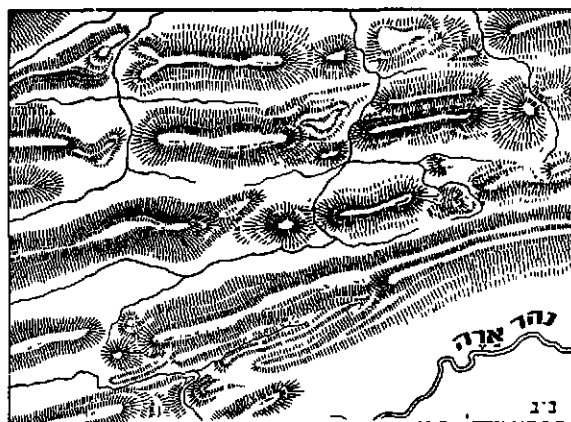
פורמולוגיה של הרילועה (שווייץ) (כל סור הוא אנטיסילניה, כל עמק — סינקלינה; נחלי-הרוחב הוצים את האנטיסילניות כנאיות צרים; נחלי-האורך הם סינקלינאליים; רשת-הנחלים ישרת-זוויות)
